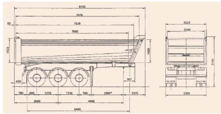
Semiremolque basculante 3 ejes
